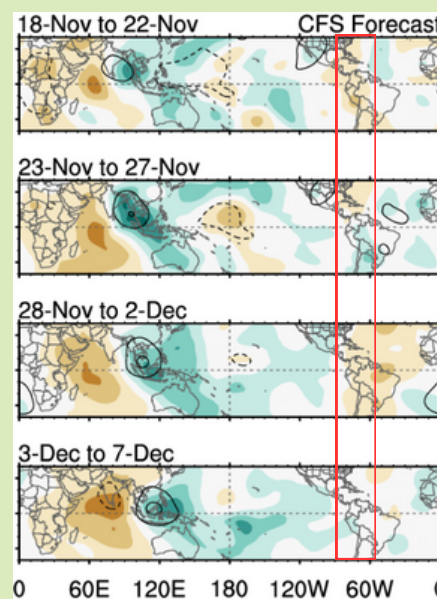
Figura 3. Pronóstico OMJ NOAA-CPC. Fuente: NOAA-CPC publicado el 17 de noviembre 2025
