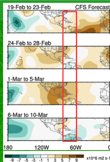
Figura 3. Pronóstico de la MJO
